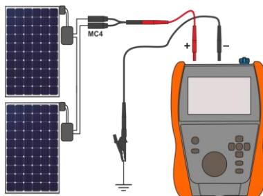
Pomiar R_{iso} w instalacji PV wyposażonej w optymalizatory
