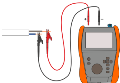
Standardowy pomiar R_{iso}
